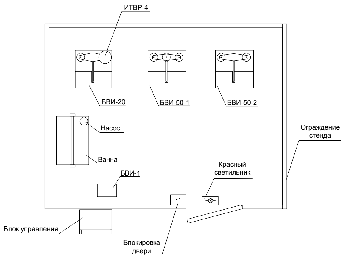
Рис. Б1 Схема размещения оборудования аппарата АВ-50/70-3
